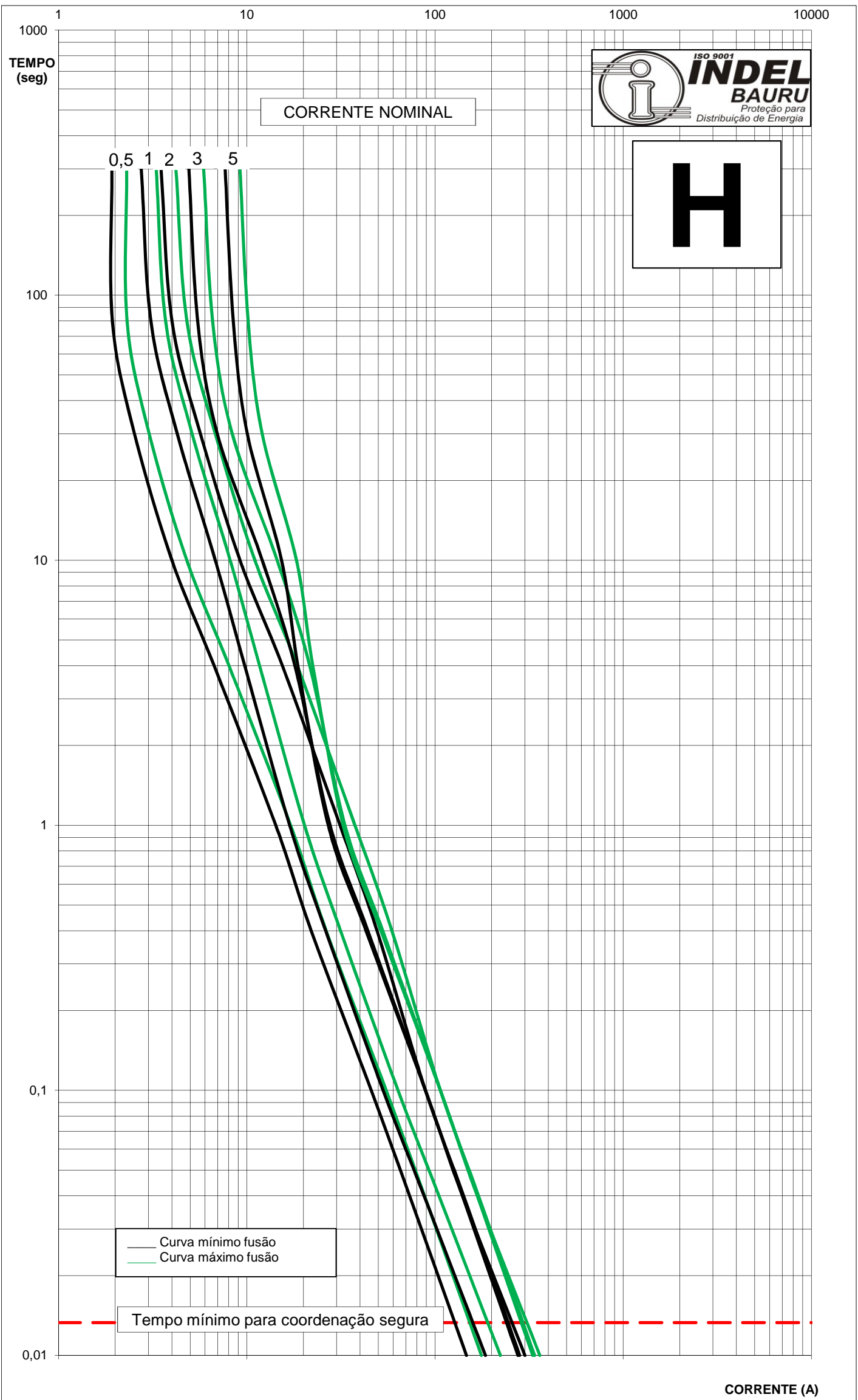
CURVAS CARACTERÍSTICAS DE FUSÃO TEMPO X CORRENTE TIPO "H" EM CONFORMIDADE COM A NORMA ABNT NBR 7282 DATA: 08/12
