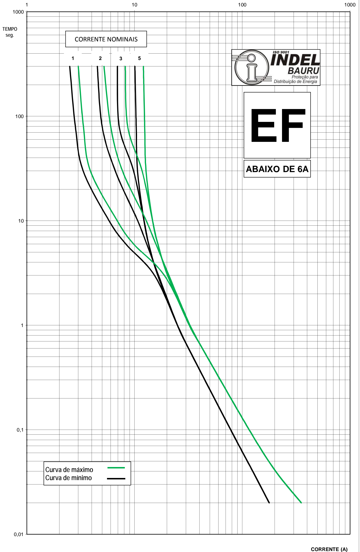
CURVAS CARACTERÍSTICAS DE FUSÃO TEMPO x CORRENTE ELOS TIPO "EF" - BASEADOS NA NORMA NEMA PUB SG2 1954 DATA: 12/96
