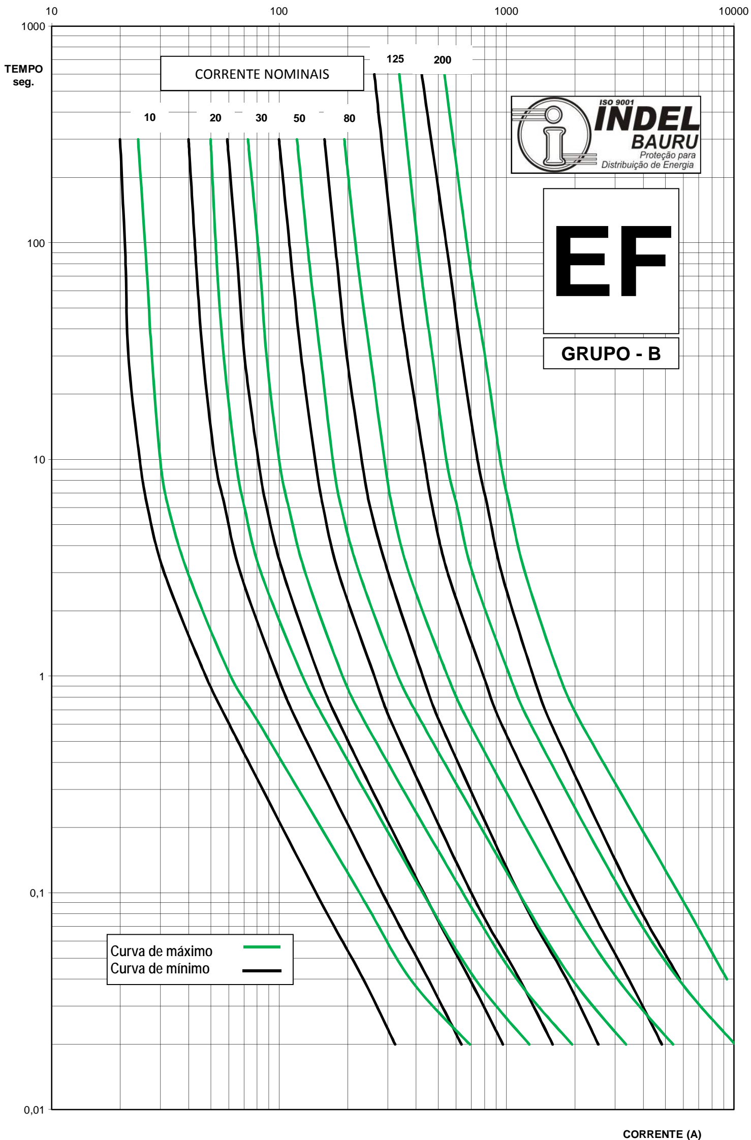
CURVAS CARACTERISTICAS DE FUSÃO TEMPO x CORRENTE ELOS TIPO "EF" - BASEADOS NA NEMA PUB SG 2 - 1954 DATA: 12/96
