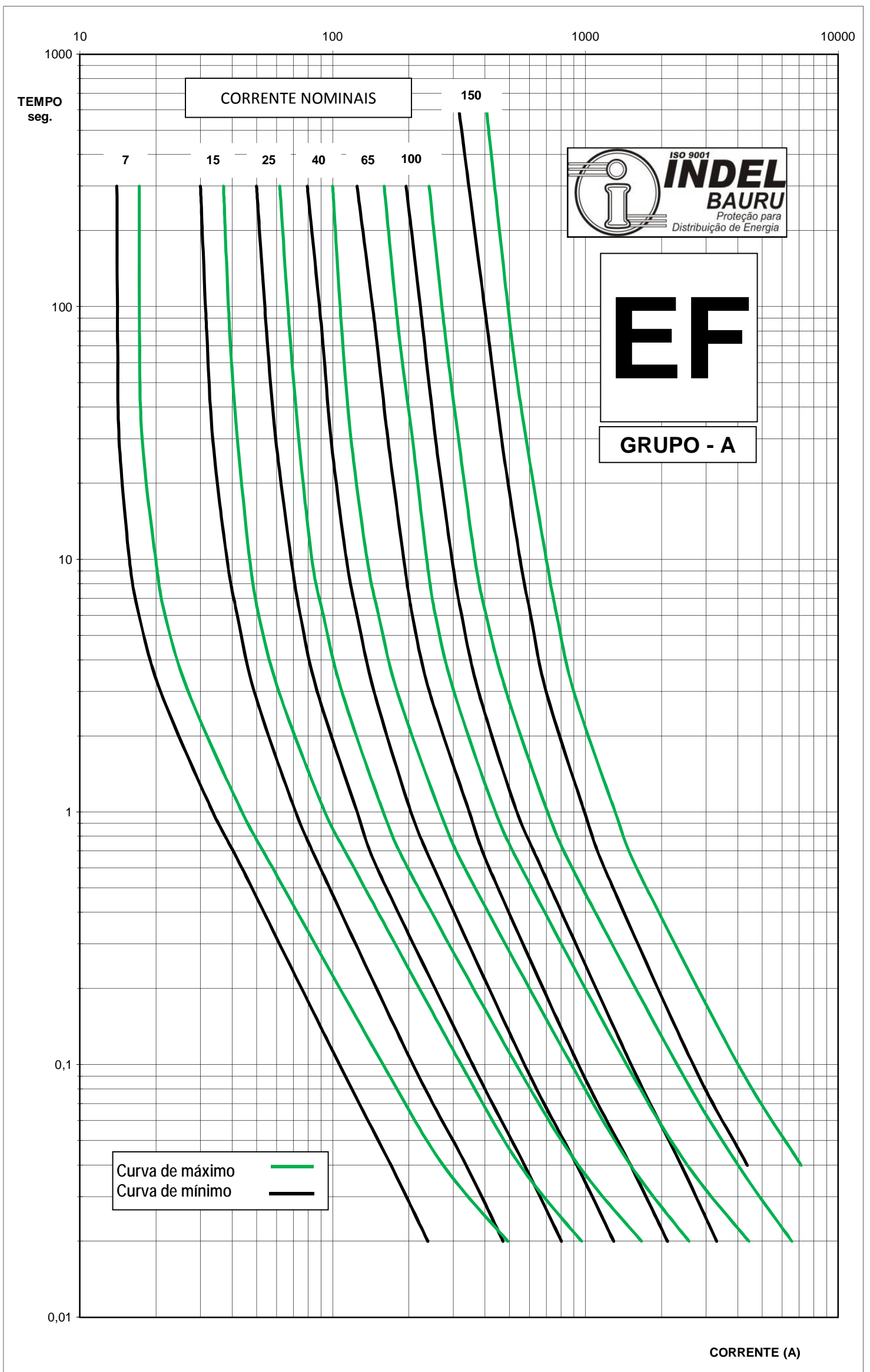
CURVAS CARACTERISTICAS DE FUSÃO TEMPO x CORRENTE ELOS TIPO "EF" - BASEADOS NA NEMA PUB SG 2 - 1954 DATA: 12/96
