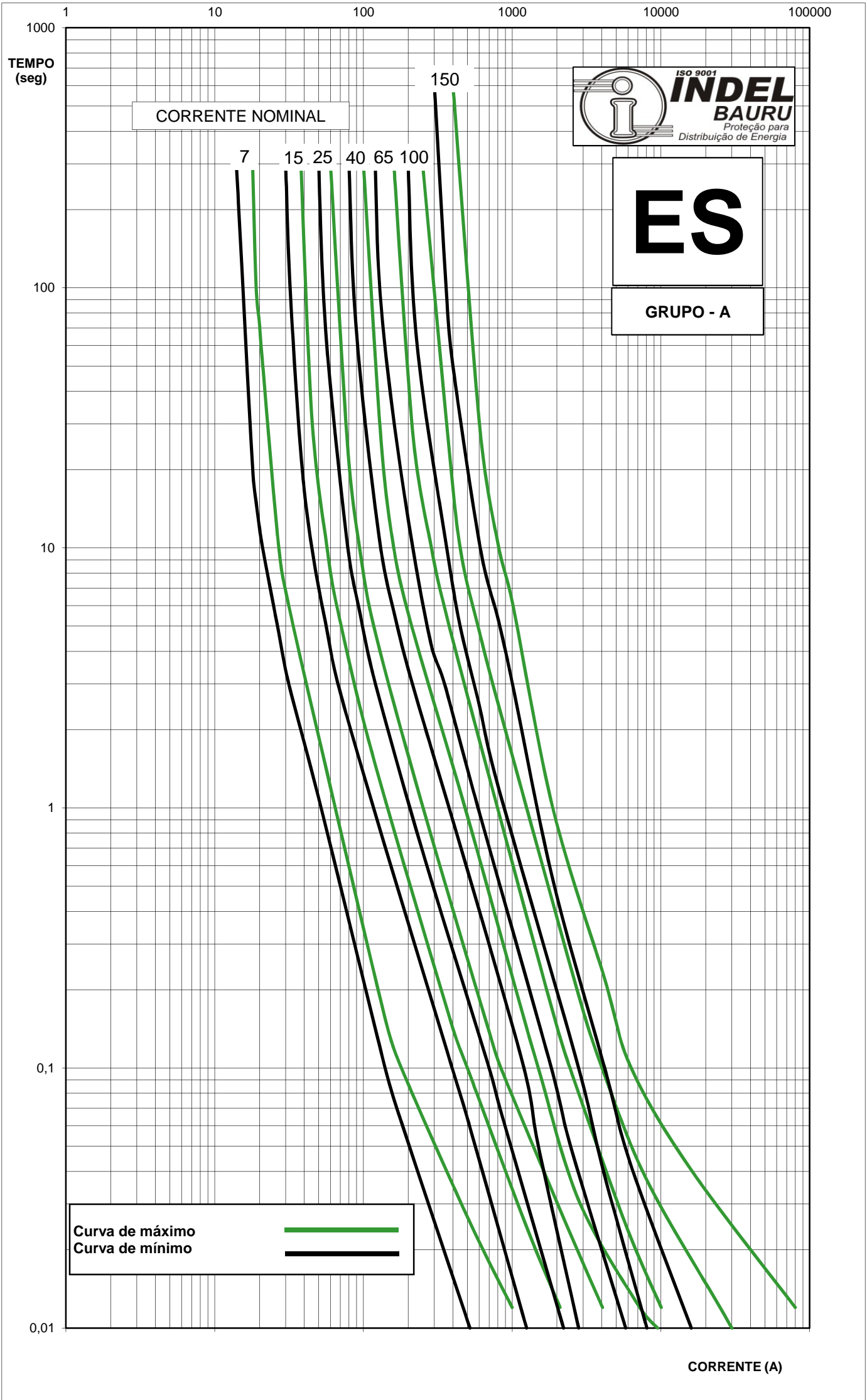
CURVAS CARACTERÍSTICAS DE FUSÃO TEMPO X CORRENTE TIPO "ES" - BASEADA NA NEMA PUB SG 2 - 1954 DATE: 12/96
