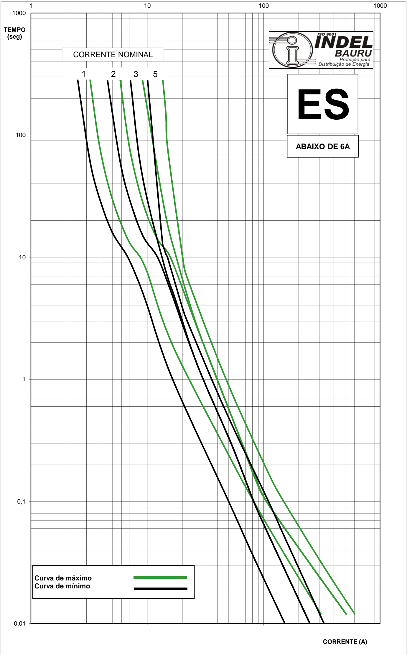
CURVAS CARACTERÍSTICAS DE FUSÃO TEMPO X CORRENTE TIPO "ES" - BASEADOS NA NEMA PUB SG 2 - 1954 DATE: 12/96
