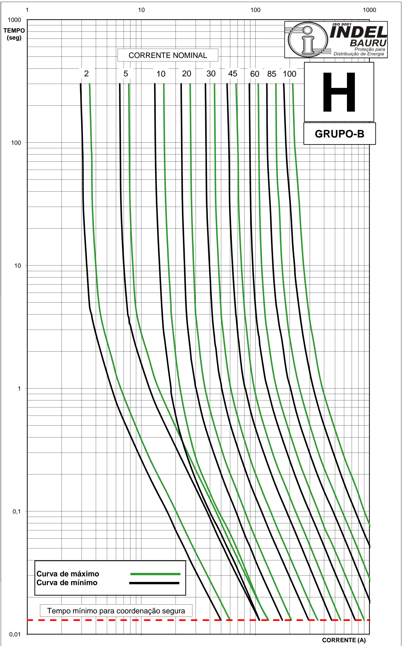
CURVAS CARACTERÍSTICAS DE FUSÃO TEMPO X CORRENTE TIPO "H NEMA" - EM CONFORMIDADE COM A NORMA NEMA PUB SG2 1954 DATE: 09/02
