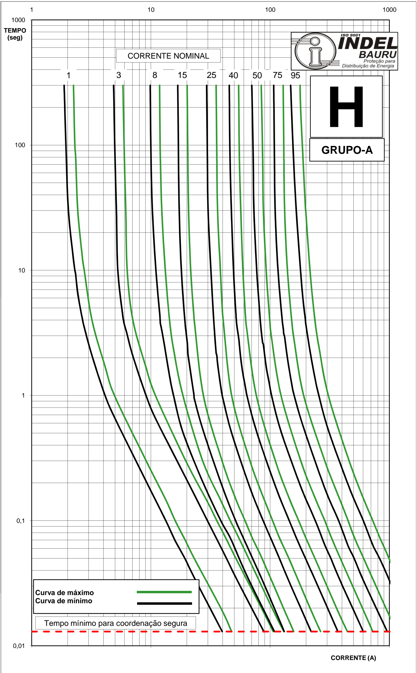
CURVAS CARACTERÍSTICAS DE FUSÃO TEMPO X CORRENTE TIPO "H NEMA" - EM CONFORMIDADE COM A NORMA NEMA PUB SG2 1954 DATE: 09/02
