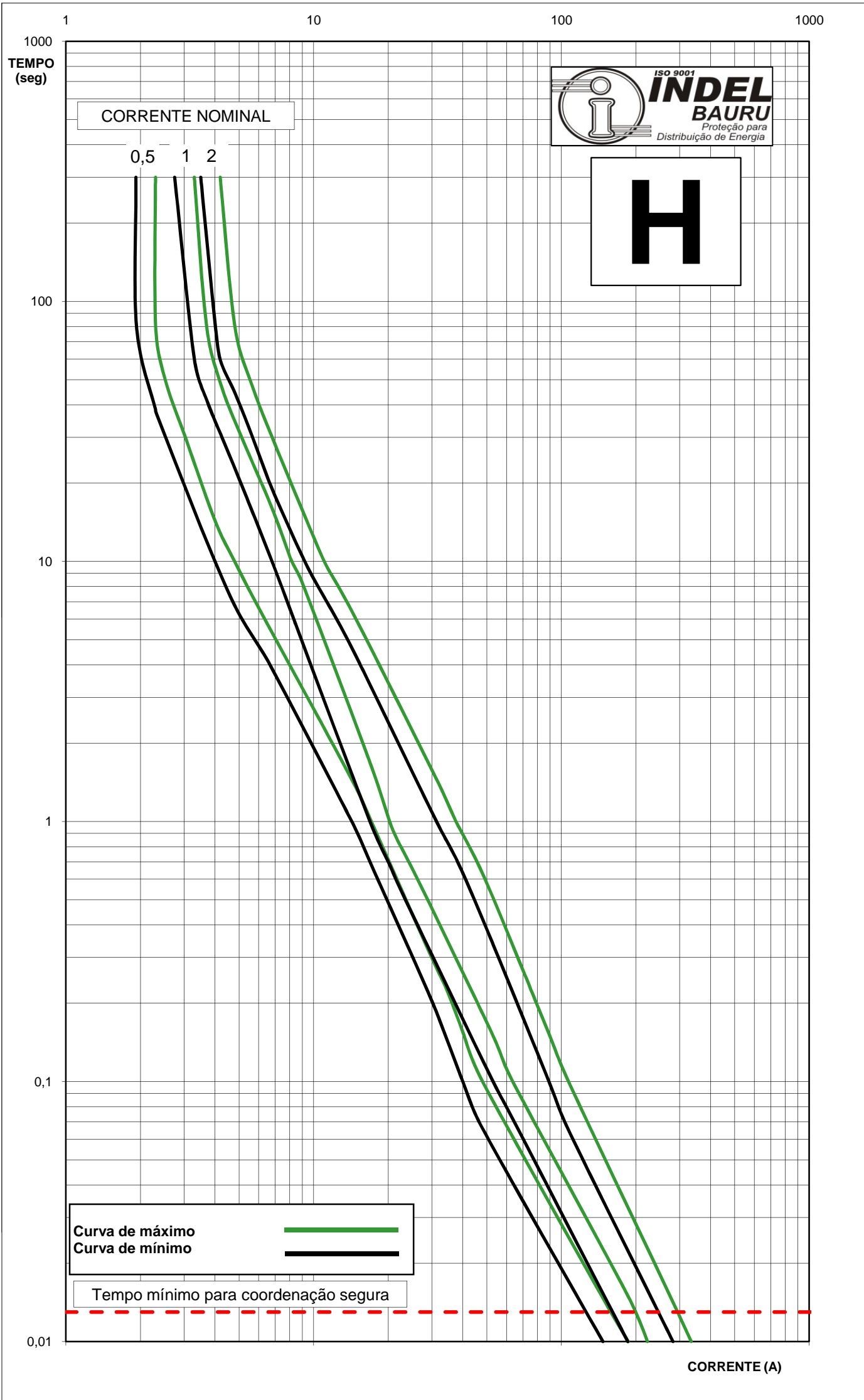
CURVAS CARACTERÍSTICAS DE FUSÃO TEMPO X CORRENTE TIPO "H OLHAL" - EM CONFORMIDADE COM A NORMA NBR 5359 DATE: 09/02
