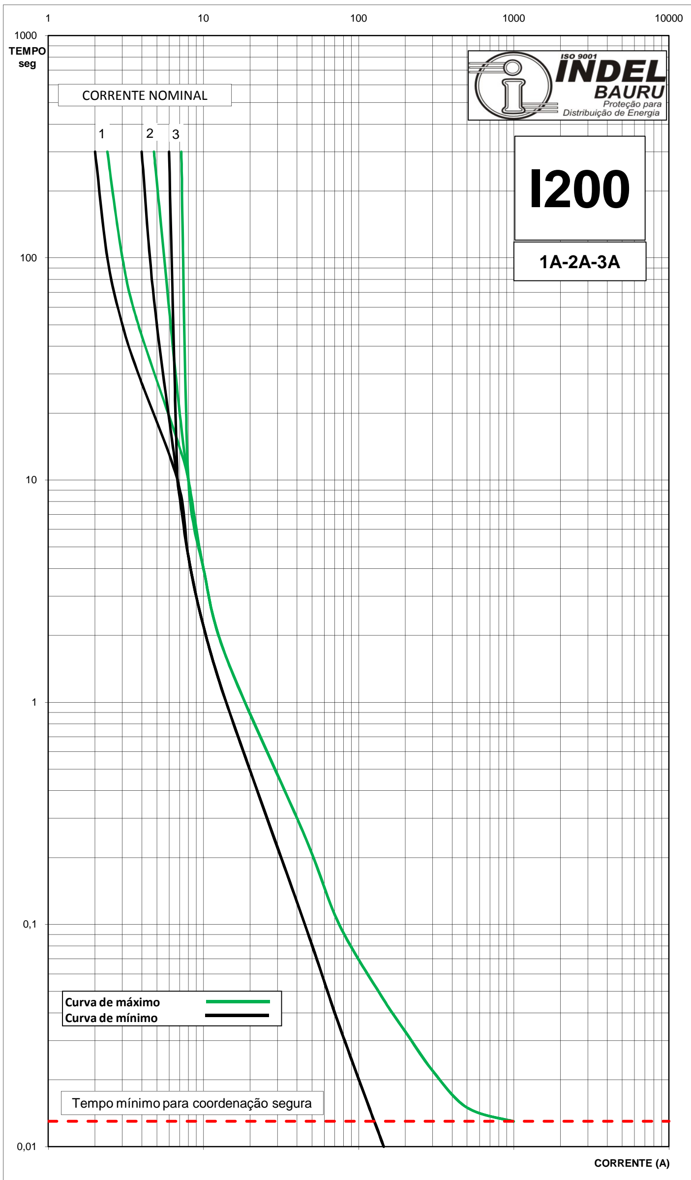
CURVAS CARACTERÍSTICAS DE FUSÃO TEMPO X CORRENTE TIPO "I200" - EM CONFORMIDADE COM A NORMA ANSI C34.42-1996 DATA: 05/10
