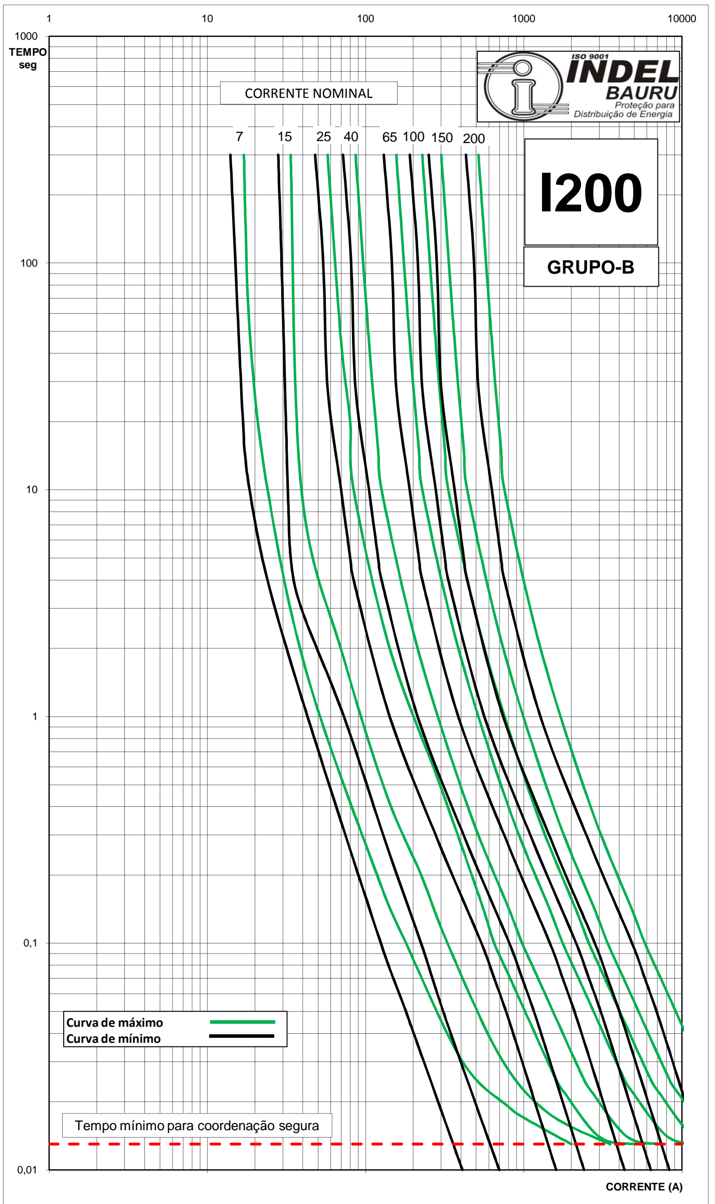
CURVAS CARACTERÍSTICAS DE FUSÃO TEMPO X CORRENTE TIPO "I200" - EM CONFORMIDADE COM A NORMA ANSI C34.42-1996 DATA: 05/10
