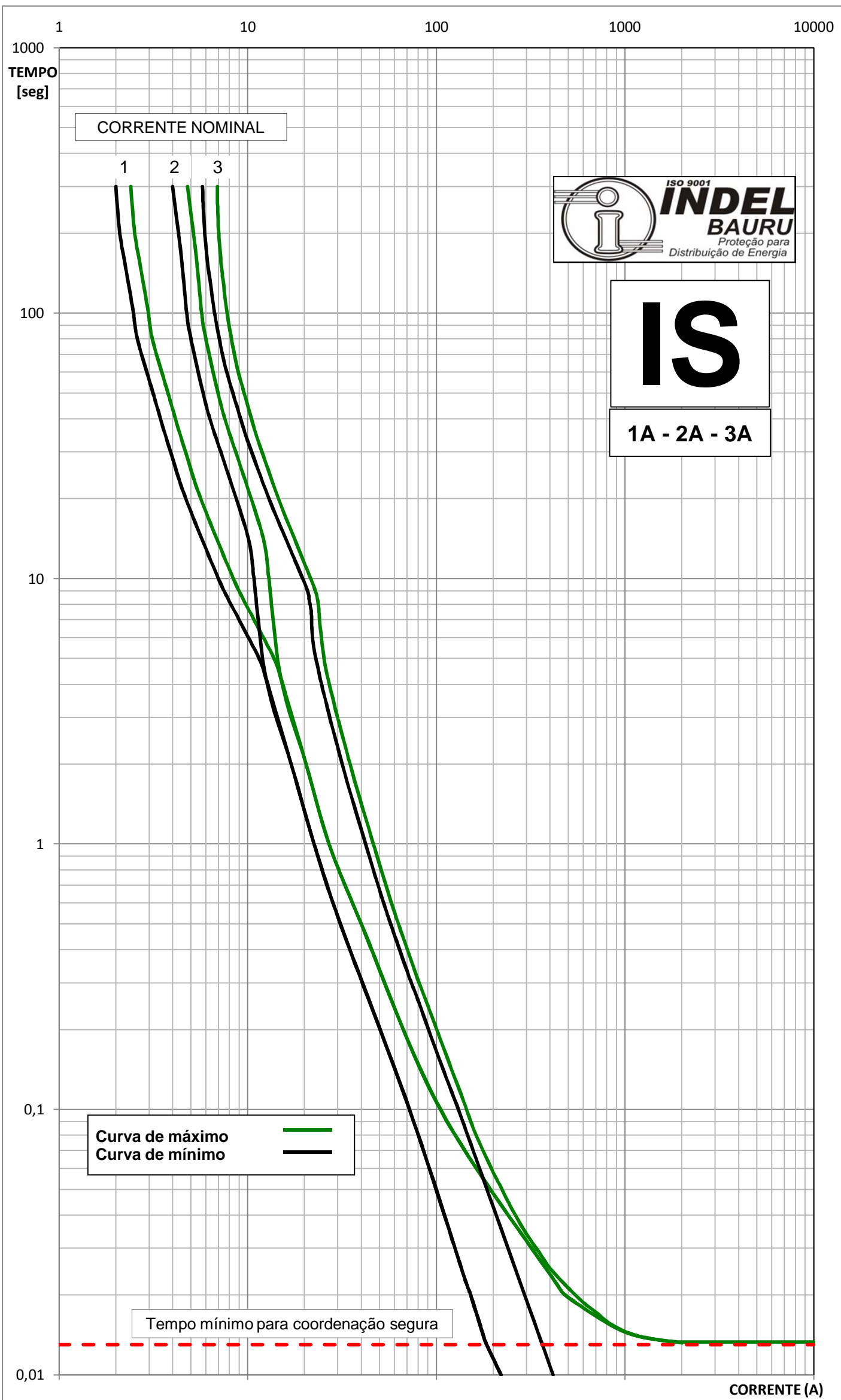
CURVAS CARACTERÍSTICAS DE FUSÃO TEMPO X CORRENTE TIPO "IS" - EM CONFORMIDADE COM A NORMA ANSI C37.42-1996 DATE: 09/02
