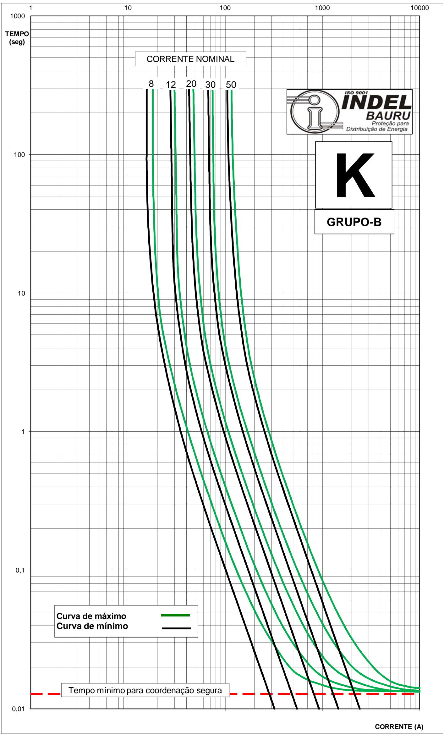
CURVAS CARACTERÍSTICAS DE FUSÃO TEMPO X CORRENTE TYPE "K OLHAL" - EM CONFORMIDADE COM A NORMA ANSI C37.42-1996 DATE: 09/02
