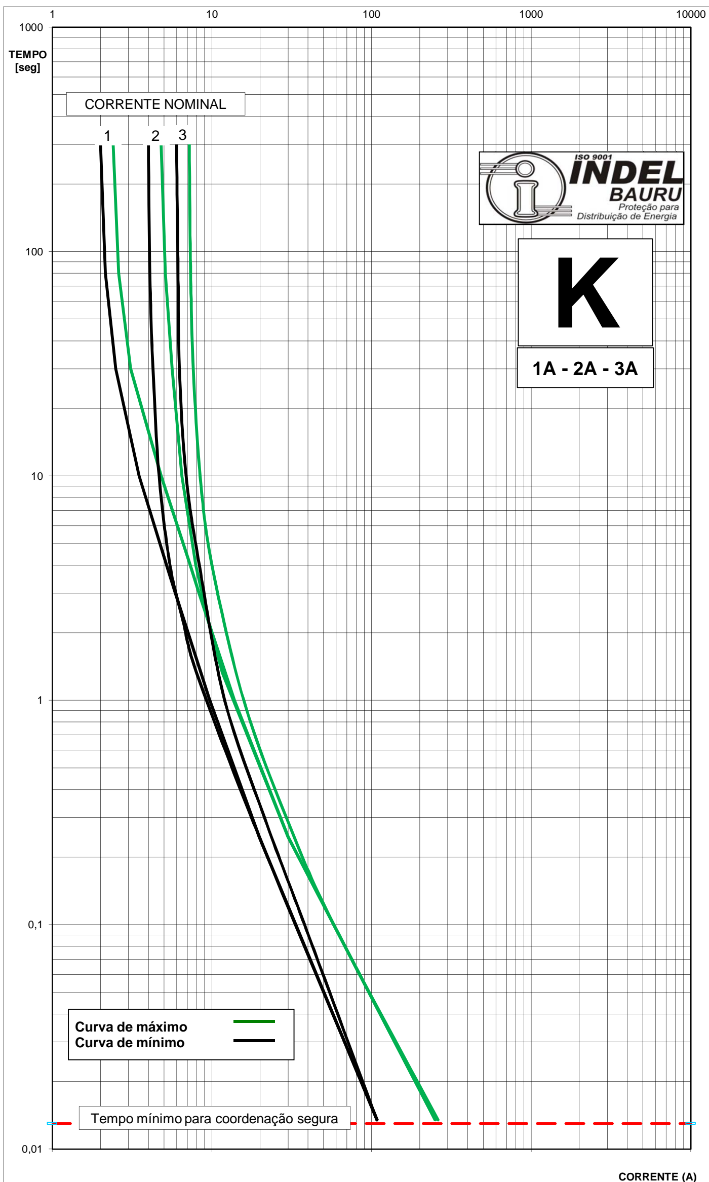
CURVAS CARACTERÍSTICAS DE FUSÃO TEMPO X CORRENTE TIPO "K OLHAL" - EM CONFORMIDADE COM A NORMA ANSI C37.42-1996 DATE: 09/02
