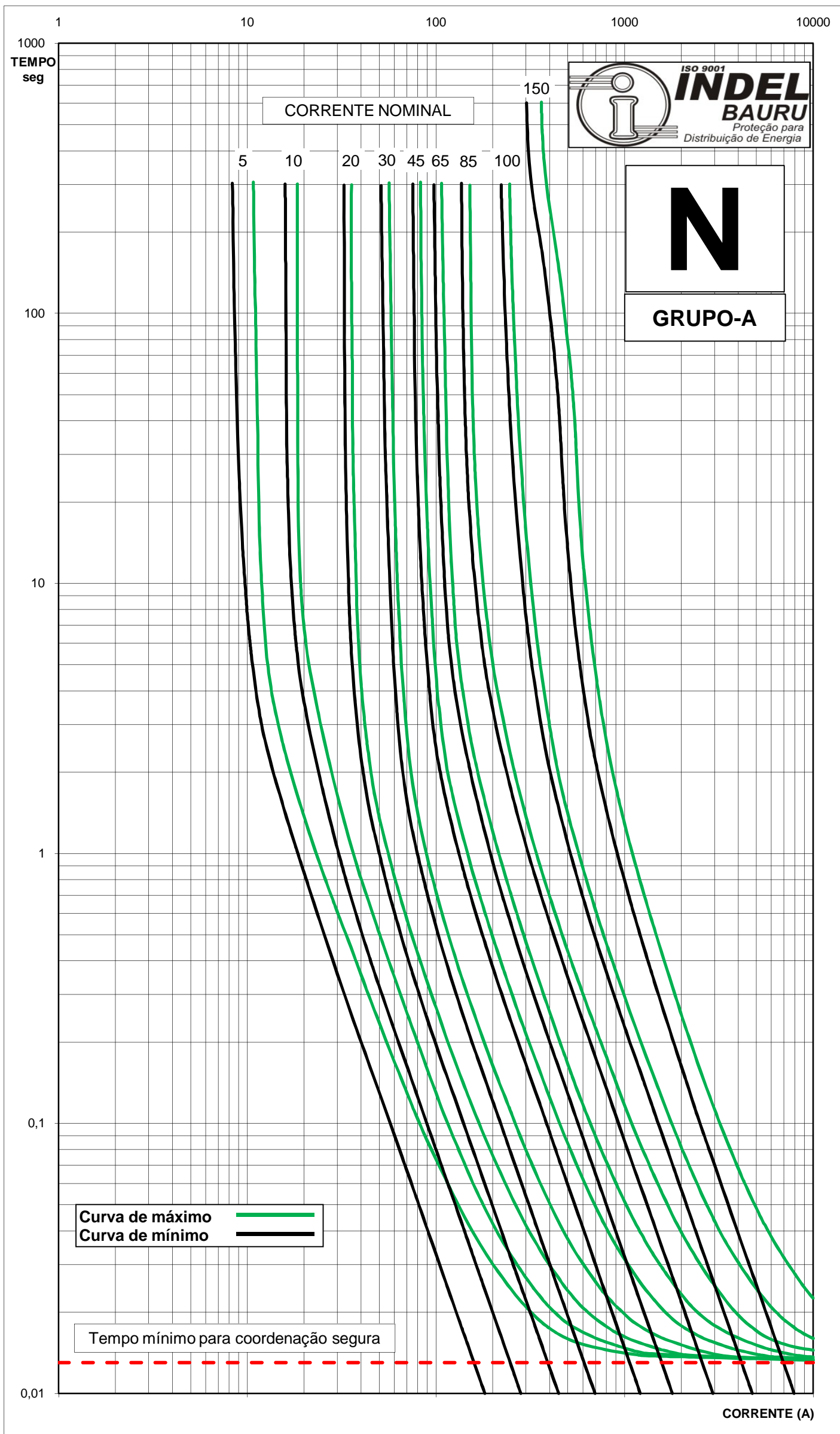
CURVAS CARACTERÍSTICAS DE FUSÃO TEMPO X CORRENTE TIPO "N" - EM CONFORMIDADE COM A NORMA ANSI C37.42-1996 DATE: 09/02
